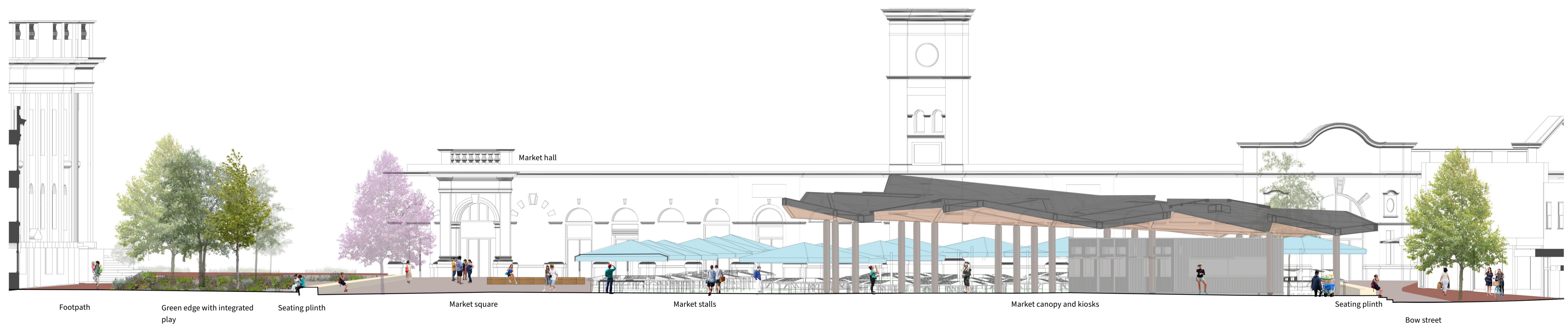
2 Section Elevation B-B Scale: 1:150
